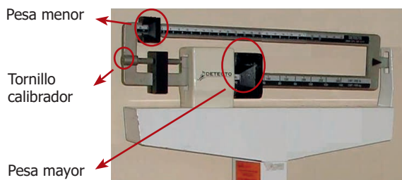
Figura 1 Parte superior de una balanza de plataforma sin tallímetro
